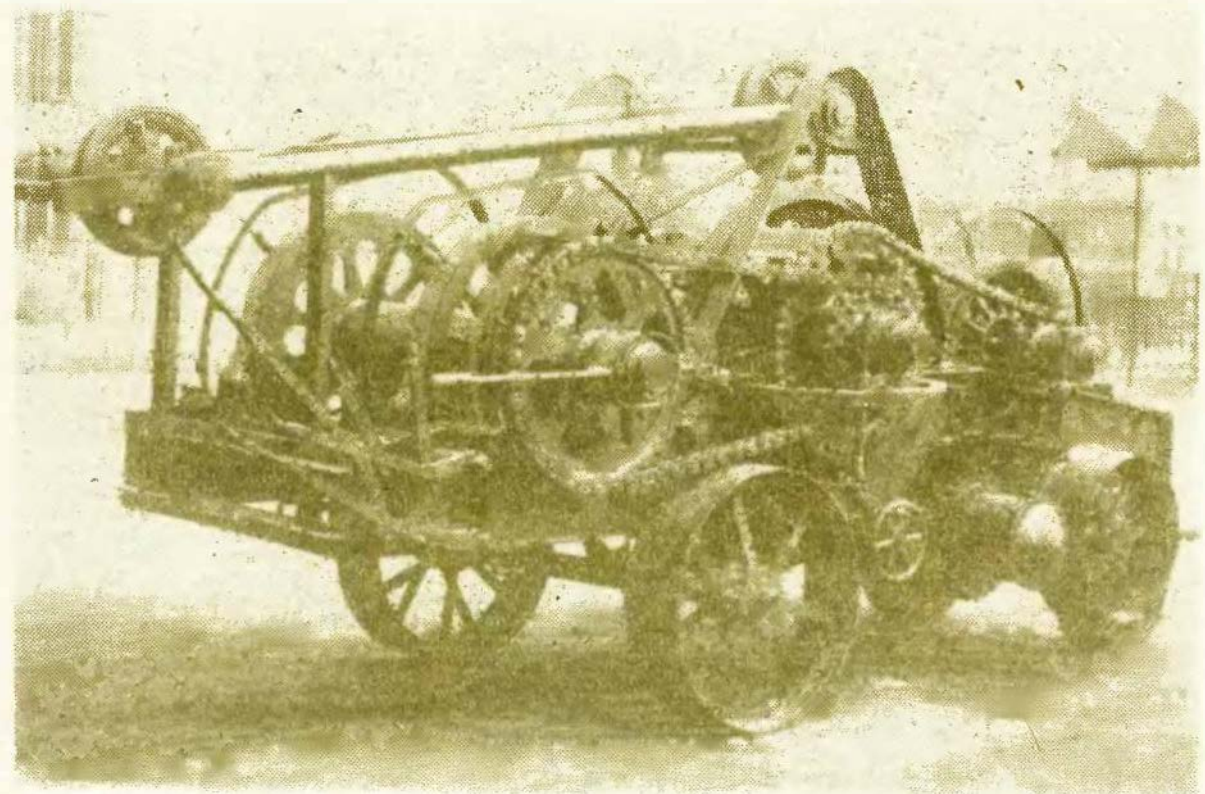
Wiertnica udarowa SMFM — wyprodukowana w 1948 r.
